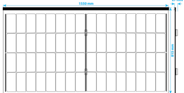
système de montage Smart BIPV - vue frontale:
