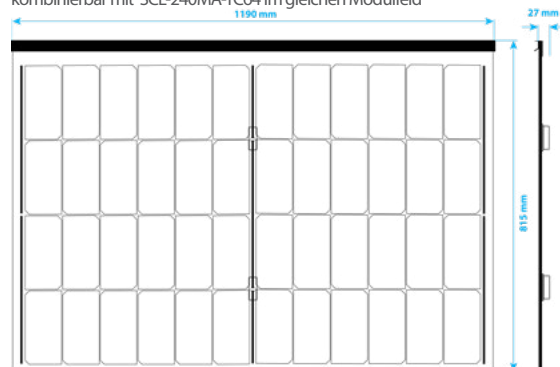
Smart BIPV Montagesystem - Frontansicht:
