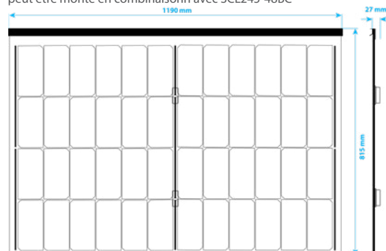
système de montage Smart BIPV - vue frontale:
