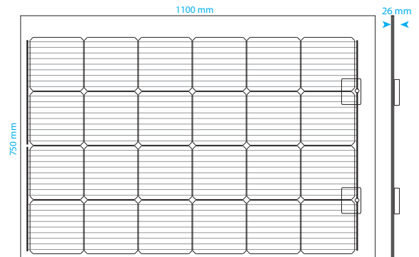
Système de montage Smart BIPV - Vue frontale:
